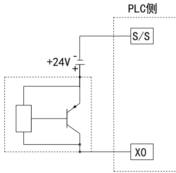
两线制（PNP 型）接近开关接线图示例
