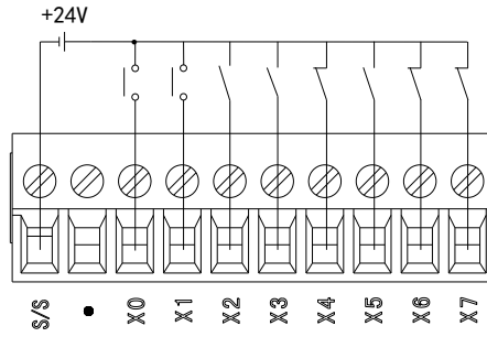
开关按钮接线图示例
