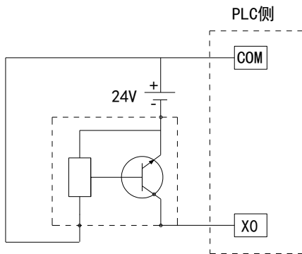
三线制 (NPN 型) 接近开关接线图示例
