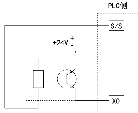
两线制 (NPN 型) 接近开关接线图示例
