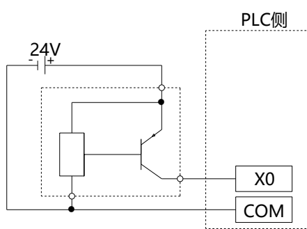
三线制 (PNP 型) 接近开关接线图示例
