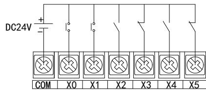
开关按钮接线图示例
