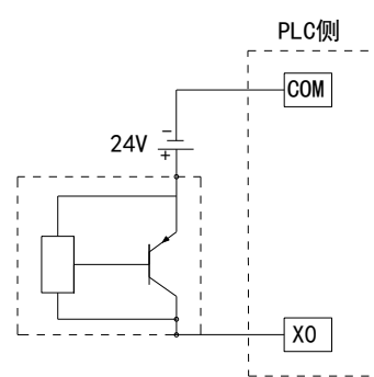
三线制 (PNP 型) 接近开关接线图示例
