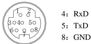
Mini Din 8 芯插座（孔）
