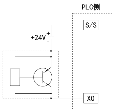
三线制 (NPN 型) 接近开关接线图示例
