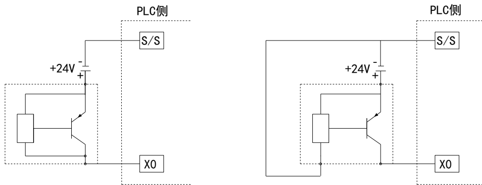
两线制（常开或常闭）接近开关接线图示例
